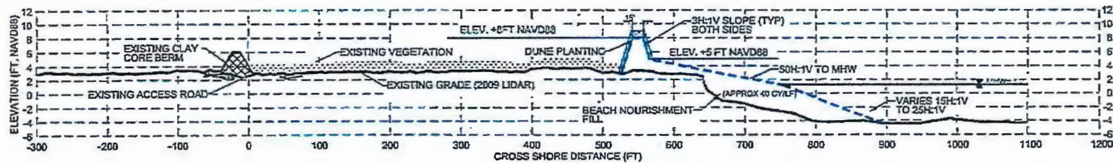
05 PROJECT SECTION STA 748+35
