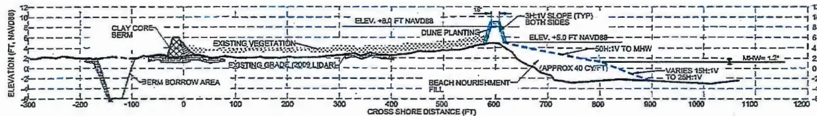
02 PROJECT SECTION STA 310+00
