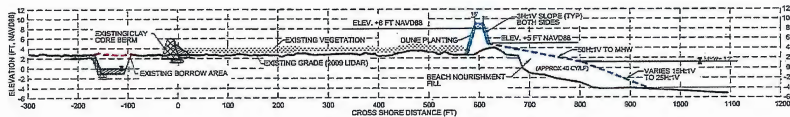
04 PROJECT SECTION STA 682+75
