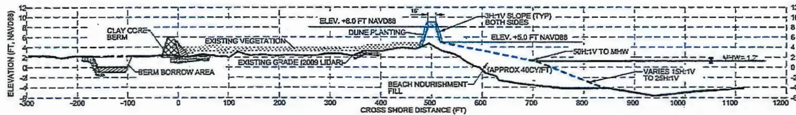
01 PROJECT SECTION STA 130+00
