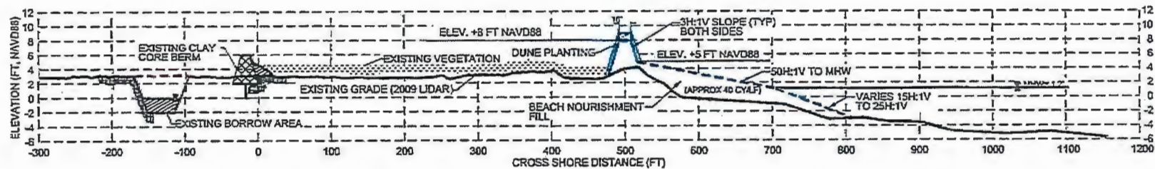
03 PROJECT SECTION STA 554+00
