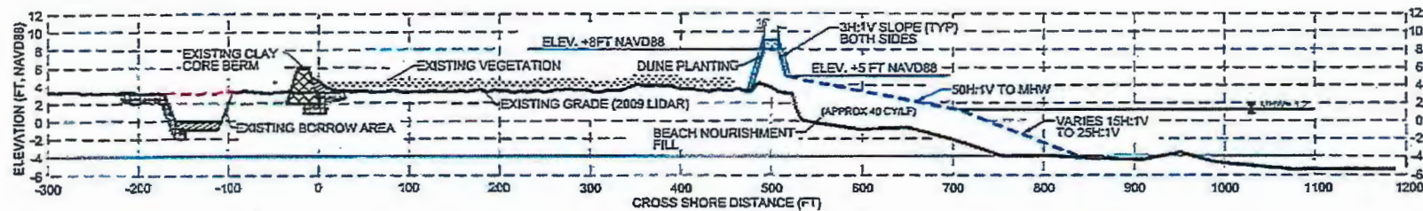
06 PROJECT SECTION STA 830+75
